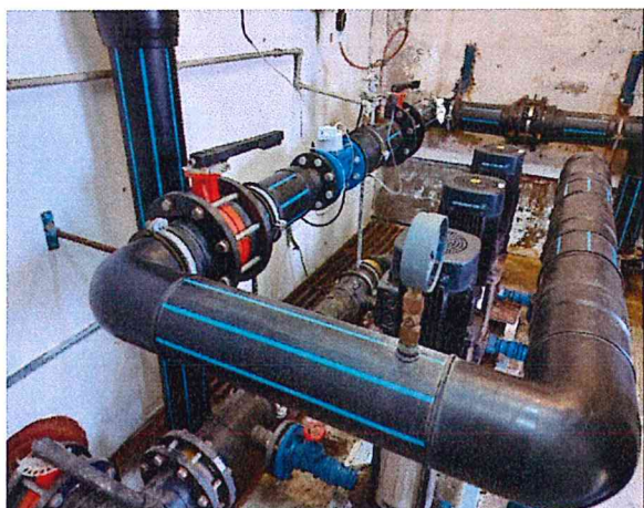
Wnętrze pomieszczenia zestawu pompowego.
